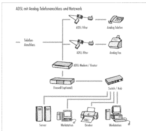
Bei einem ISDN-Anschluss spaltet ein ADSL-Splitter die Signale für das NT (Netzabschlussgerät) und für das ADSL-Modem auf. Beim Analog-Anschluss reicht das Einsetzen eines ADSL-Filters für den Anschluss des Telefons oder des Faxes. Für ein kleines Netzwerk zu Hause wird an das ADSL-Modem/Router ein Switch oder Hub angeschlossen, der die Signale an den Server, den PC oder den Drucker verteilt. (Graphik von green.ch ).
